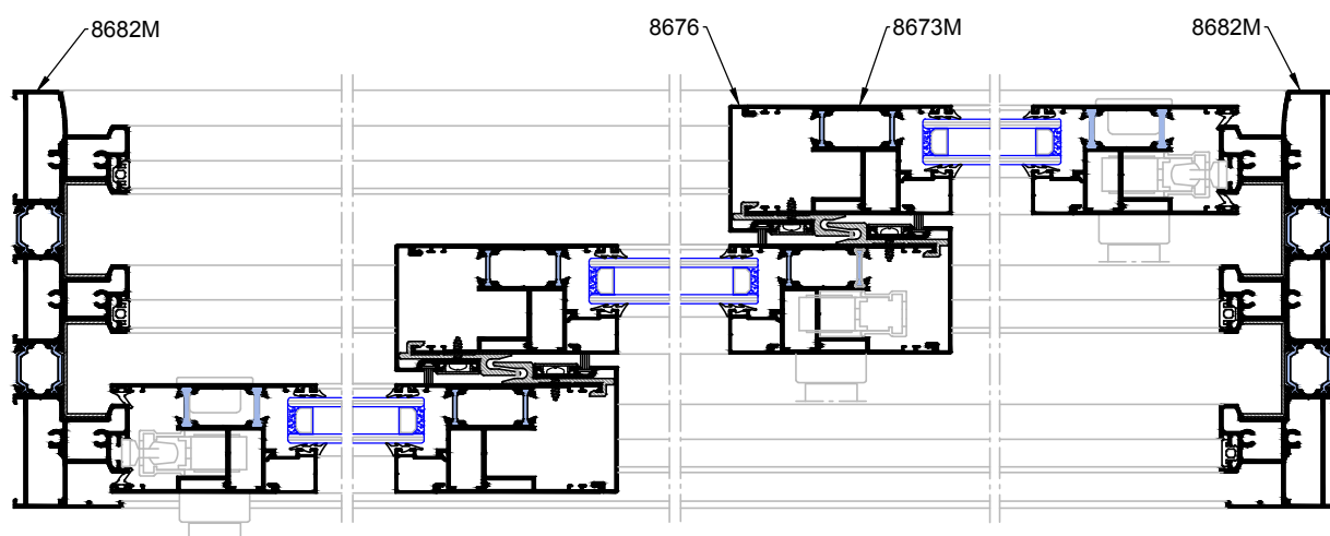
Sección A-A'
