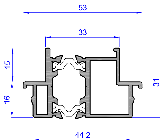
Acople 4 hojas Matra 135 RPT
