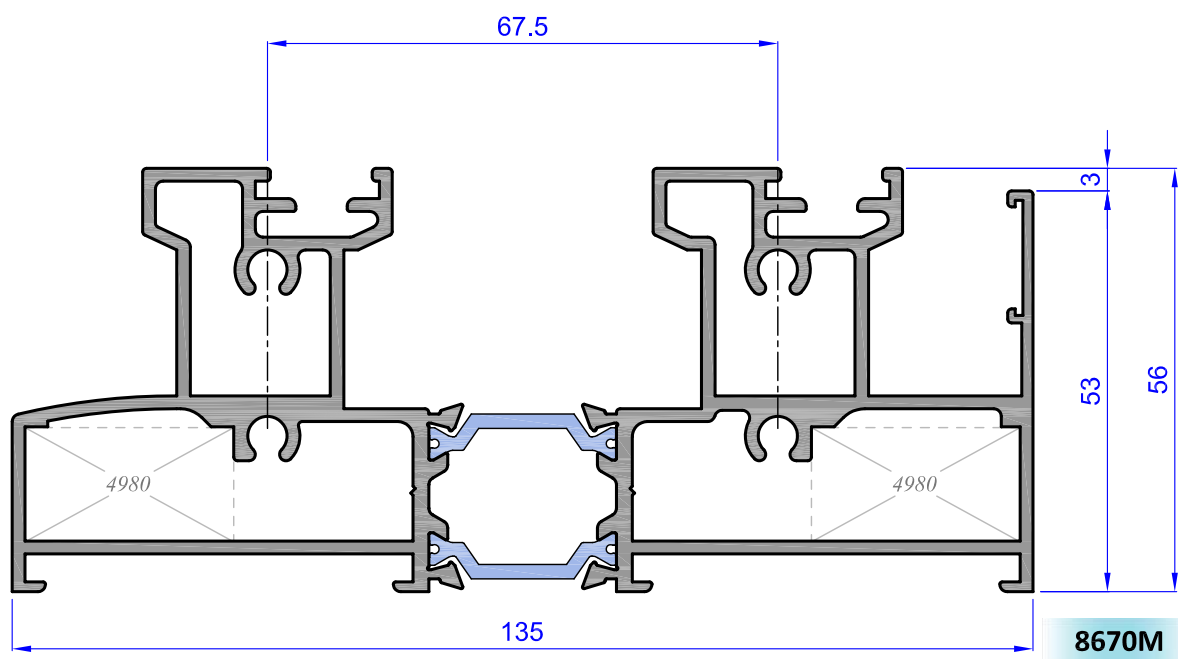
Cerco Perimetral 135 mm.
