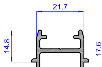
Acople hoja multipunto
