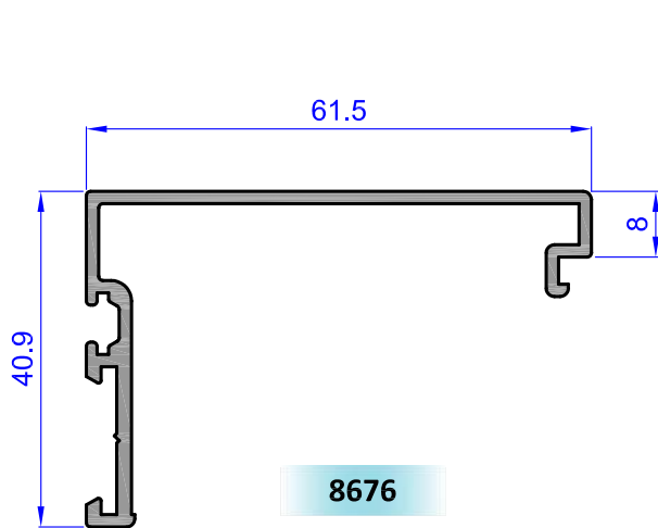
Acople central hoja
