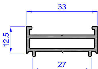
Acople cerco lateral
