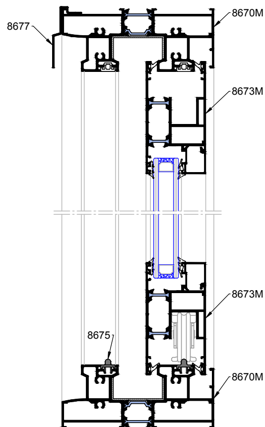
Sección B-B'
