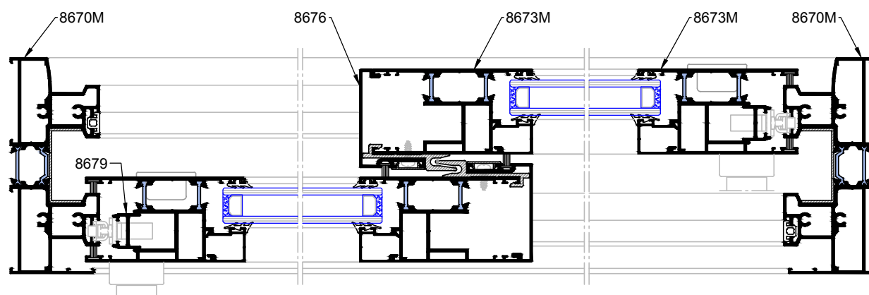
Sección A-A'
