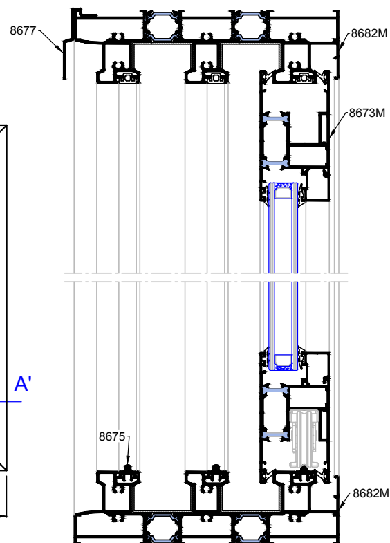
Sección B-B'
