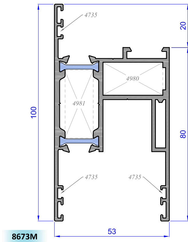
Hoja Perimetral 100 x 53 mm.
