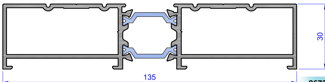
Cerco Lateral 135 mm.
