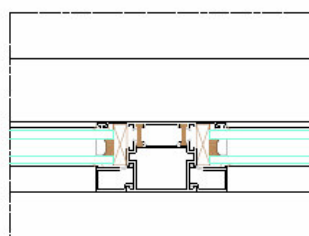
DETALLE F
